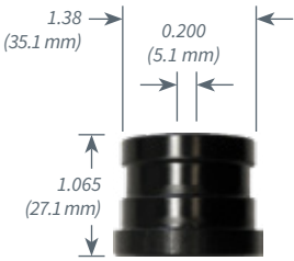
A-1LN (Delrin) A-1LN-A (Aluminum) A-1LN-LW (Large Wire) Lincoln Electric®
